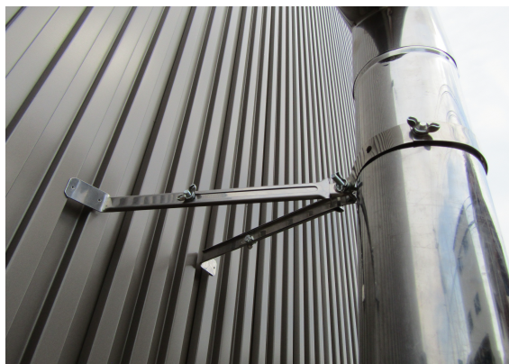
煙突支持金具 使用例
