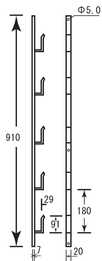
【寸法図】 (3尺用)
